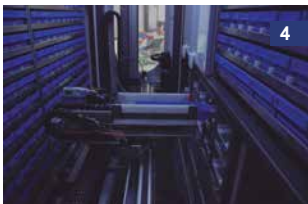
4 O braço robótico entrega o bin em uma gaveta dinâmica.
